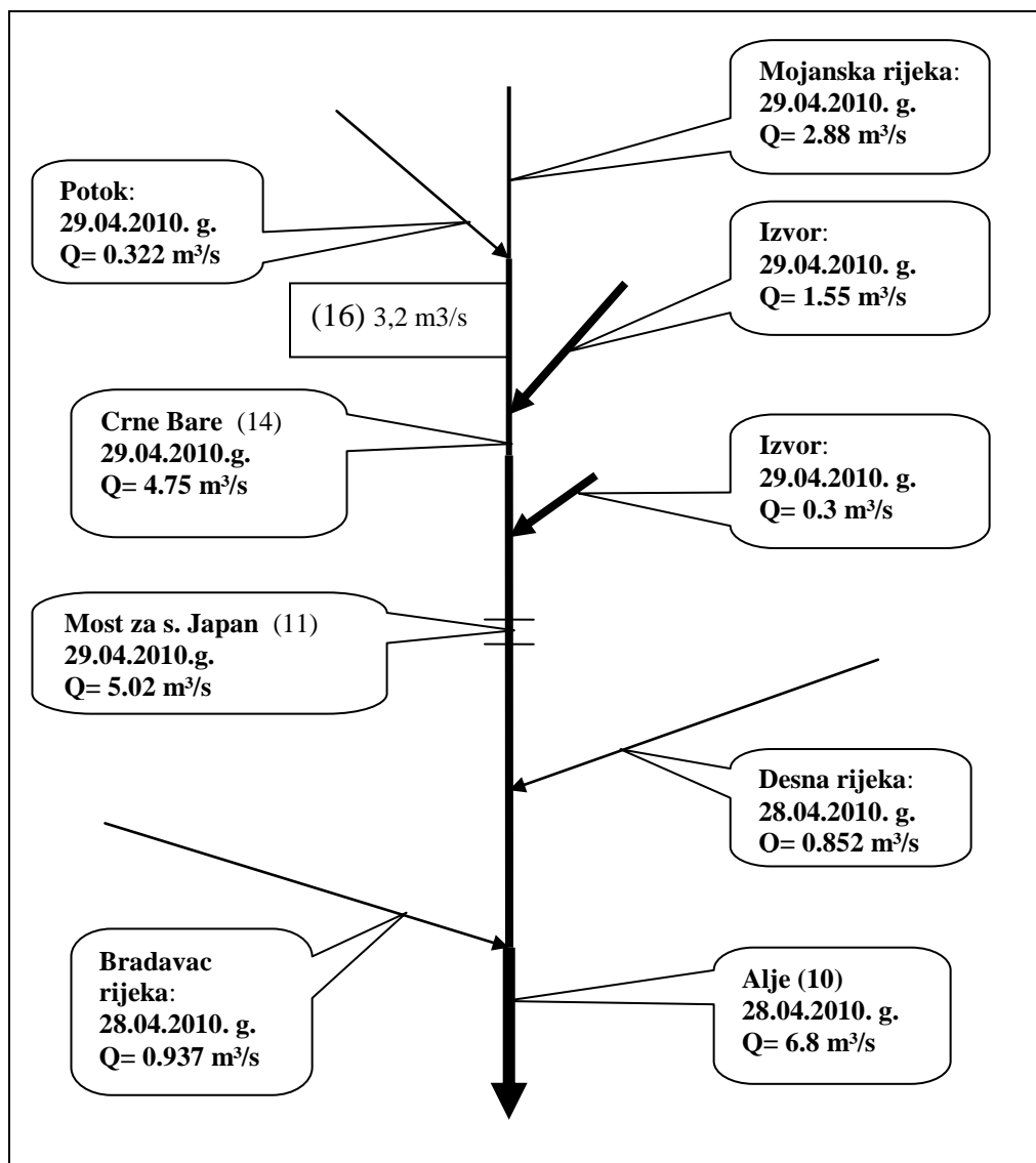
Slika 9 Pritoci na vodotoku Mojanska rijeka-Peročica-Zlorečica (u zagradi su karakteristične točke)
