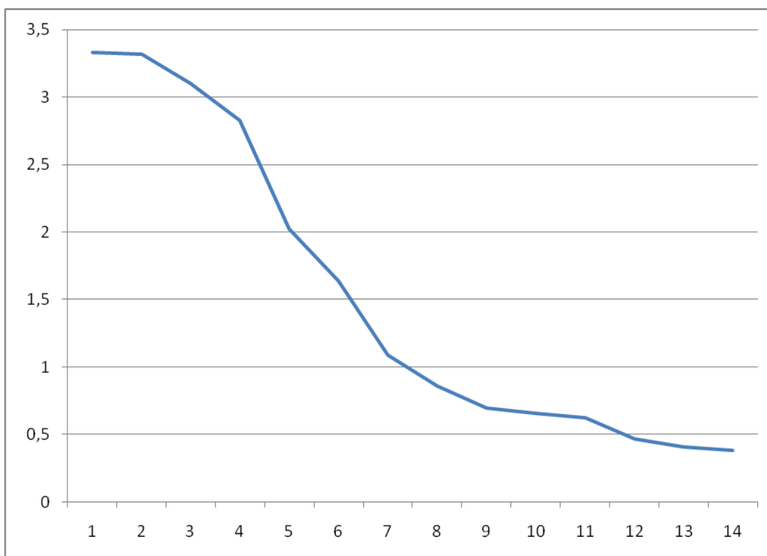
Slika 10 Razdioba protoka Mojanske rijeke (m 3 /s) na mostu Jošanica (mjerena vršena u okviru projekta Norveške Vlade u vremenu od 26.07.2007. do 28.08.2008.)
