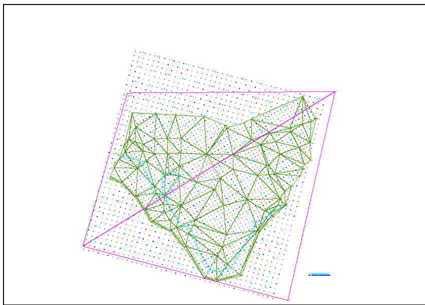
Slika 12 Oblik akumulacije Kočevi, prema [3]
